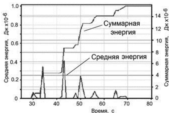
Рис. 3.20. Изменение средней энергии и суммарной энергии импульсов АЭ на стадии деформационного упрочнения образца.
