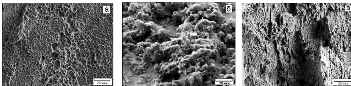
Рис. 4.17. Фрактография изломов статического растяжения образцов серии 2 после различных режимов отпуска: а – исходное состояние; б – отпуск при 400 0 С; в – отпуск при 650 0 С.
