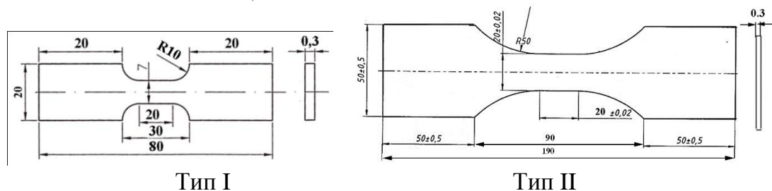
Рис. 5.16. Образцы для испытания на статическое растяжение и усталость.
