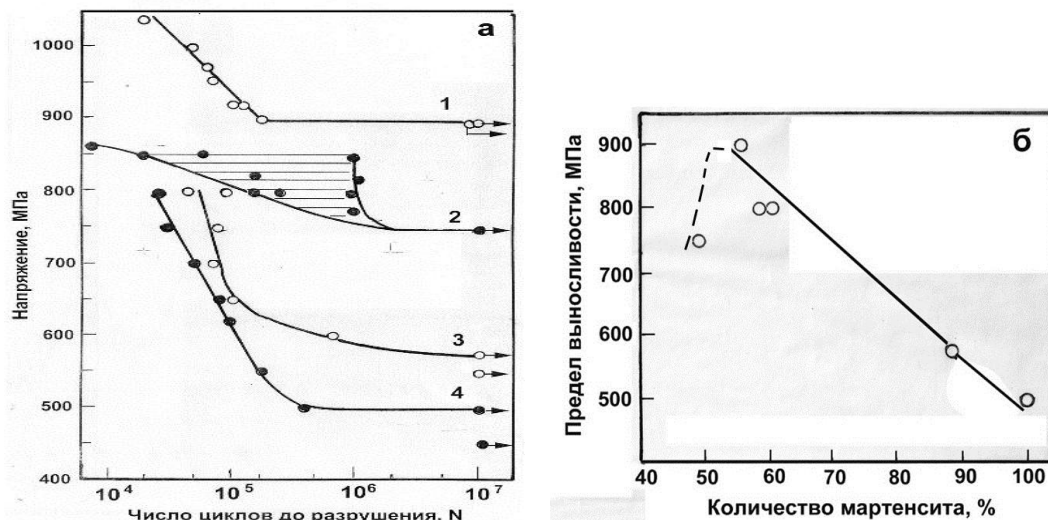
Рис. 5.10. Кривые усталости стали ВНС 9-Ш (а) и зависимость предела выносливости от количества мартенсита (б): а - 1 - партия 2; 2 – партия 1; 3 – партия 3; 4 – партия 4.
