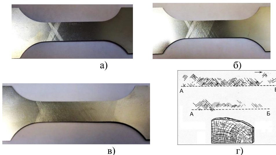
Рис. 3.17. Линии Людерса – Чернова на образцах из стали ВНС9-Ш и в опытах Людерса: а – деформация 1,7%; б – 3,4%; в – 10,75%.; -г-[48].
