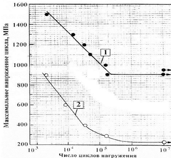
Рис. 5.15. Кривые усталости образцов из стали ВНС9 – Ш: 1 – кривая усталости без концентратора напряжений; 2 – кривая усталости с концентратором напряжений.
