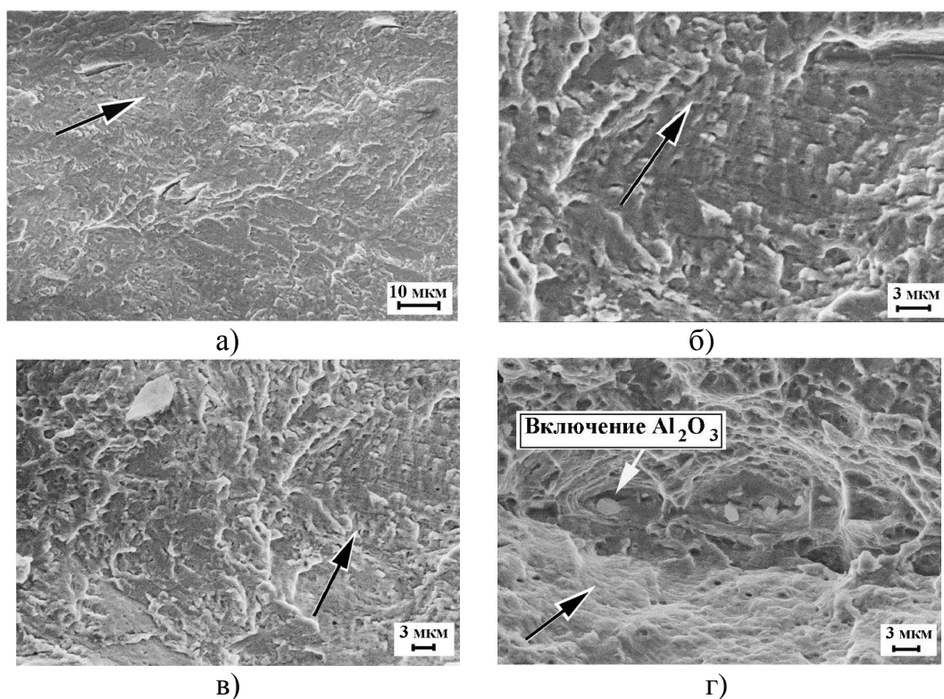
Рис. 5. 13. Фрактография усталостного разрушения образца из партии 2 исходного материала: \sigma_{\min} = 500 МПа, \sigma_{\max} = 1125 МПа, долговечность до разрушения 10^5 циклов нагружения. Стрелками указано направление распространения усталостной трещины.
