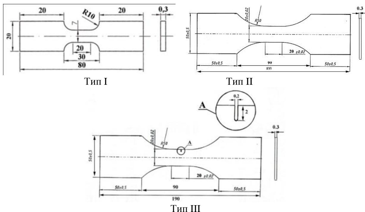
Рис. 2.1. Образцы для испытания статическое растяжение и усталость.
