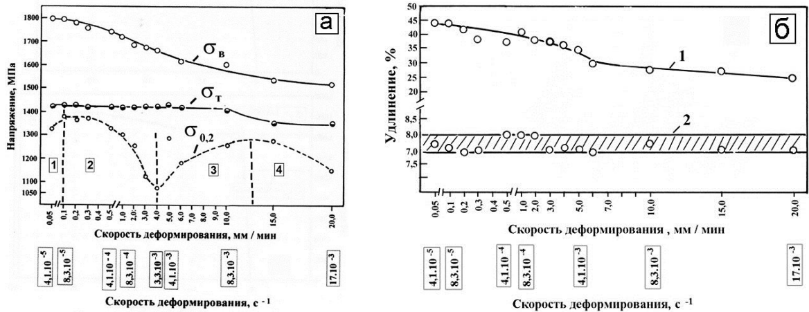
Рис.4.4. Влияние скорости деформирования на механические свойства образцов серии 1 стали ВНС9-III: а – прочностные характеристики; б – относительное удлинение \delta (1) и длина площадки текучести \epsilon_T (2).
