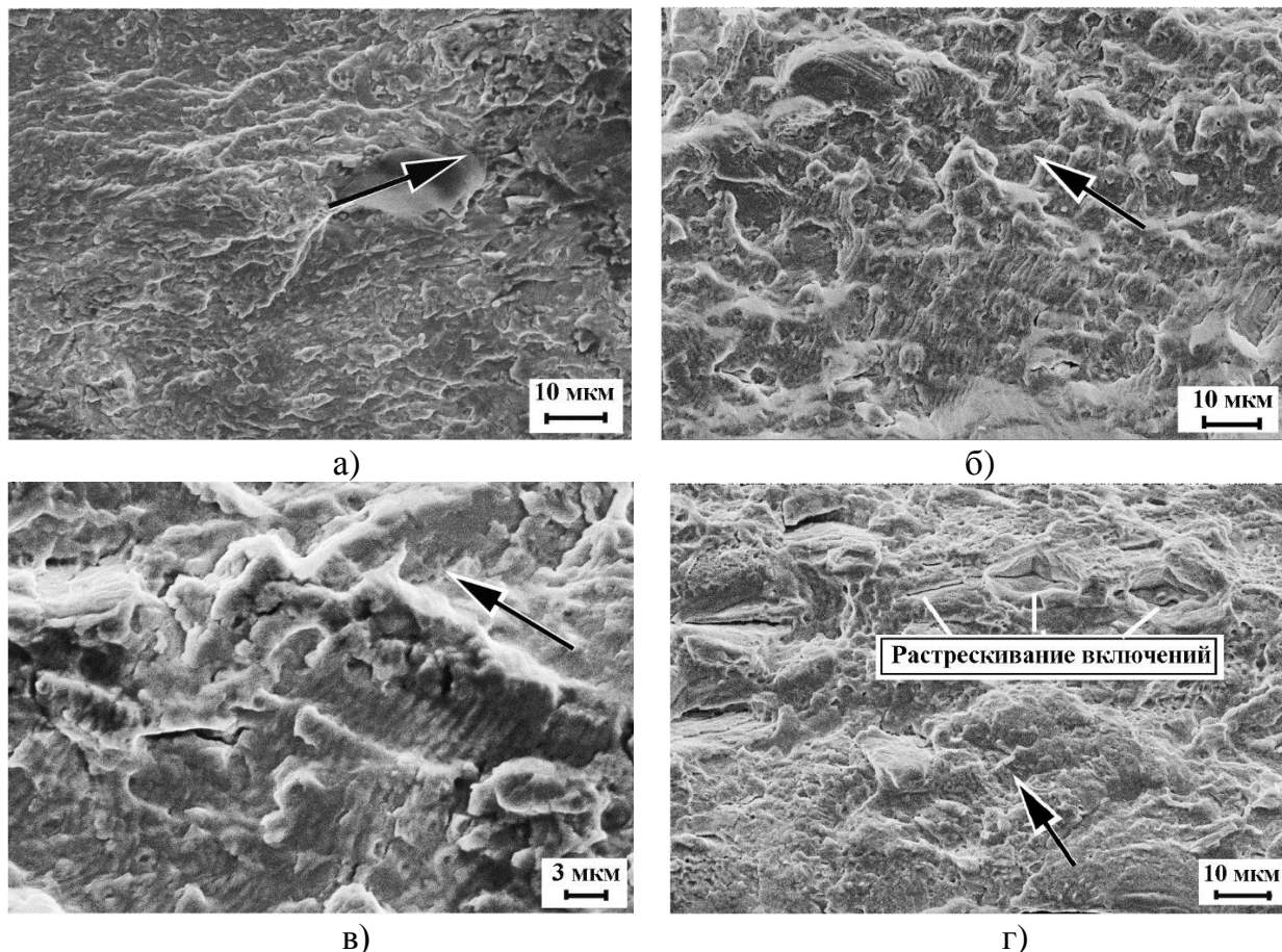
Рис. 5.12. Фрактография усталостного разрушения образца из партии 2 исходного материала: \sigma_{\min} = 100 МПа, \sigma_{\max} = 875 МПа, долговечность до разрушения 1 \cdot 10^5 циклов нагружения. Стрелками указано направление распространения усталостной трещины.
