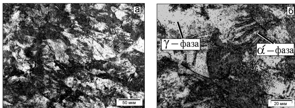
Рис. 3.1. Микроструктура стали ВНС9-Ш в исходном состоянии (оптический микроскоп).
