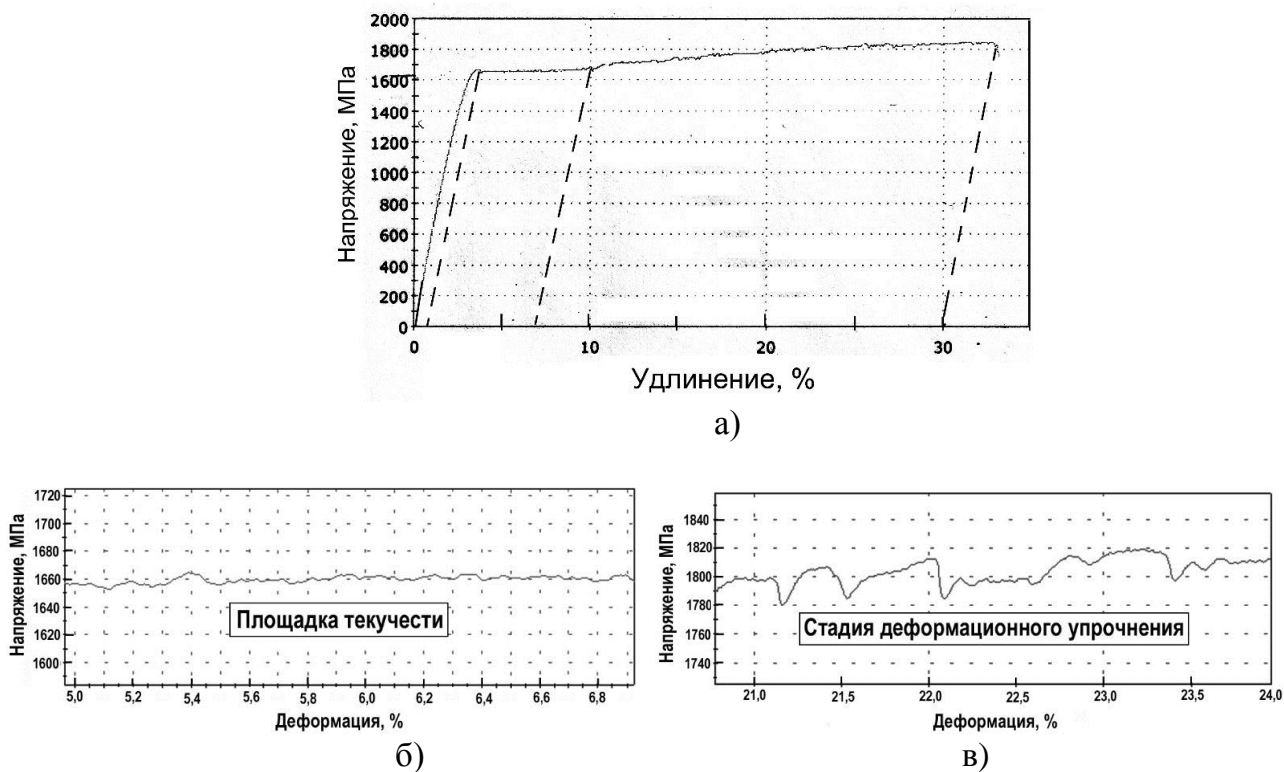
Рис. 3.13. Кривая статического растяжения образца из стали ВНС9-Ш: после удалений поверхностного слоя глубиной 20 мкм (а); более детальная картина участка кривой на стадии текучести (б) и на конечной стадии деформационного упрочнения (в).
