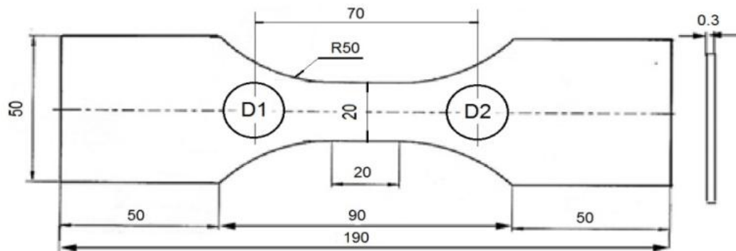
Рис. 3.20. Образец типа II для испытания на статическое растяжение (D1, D2 – места установки преобразователей АЭ).
