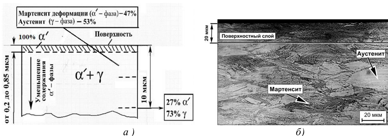
Рис. 3.11. Схема фазового состава тонколистовой трип – стали ВНС9-Ш в зависимости от удаления от поверхности материала (а) и структура исходного материала (б).
