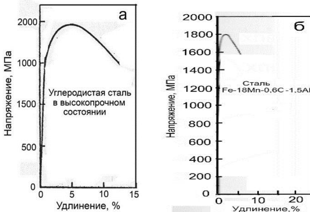
Рис. 3.15. Кривые статического растяжения углеродистой стали (0,45C) [53] (а) и высокомарганцевой твип-стали (Fe-18Mn- 0,6C-1,5 Al) [54] (б).
