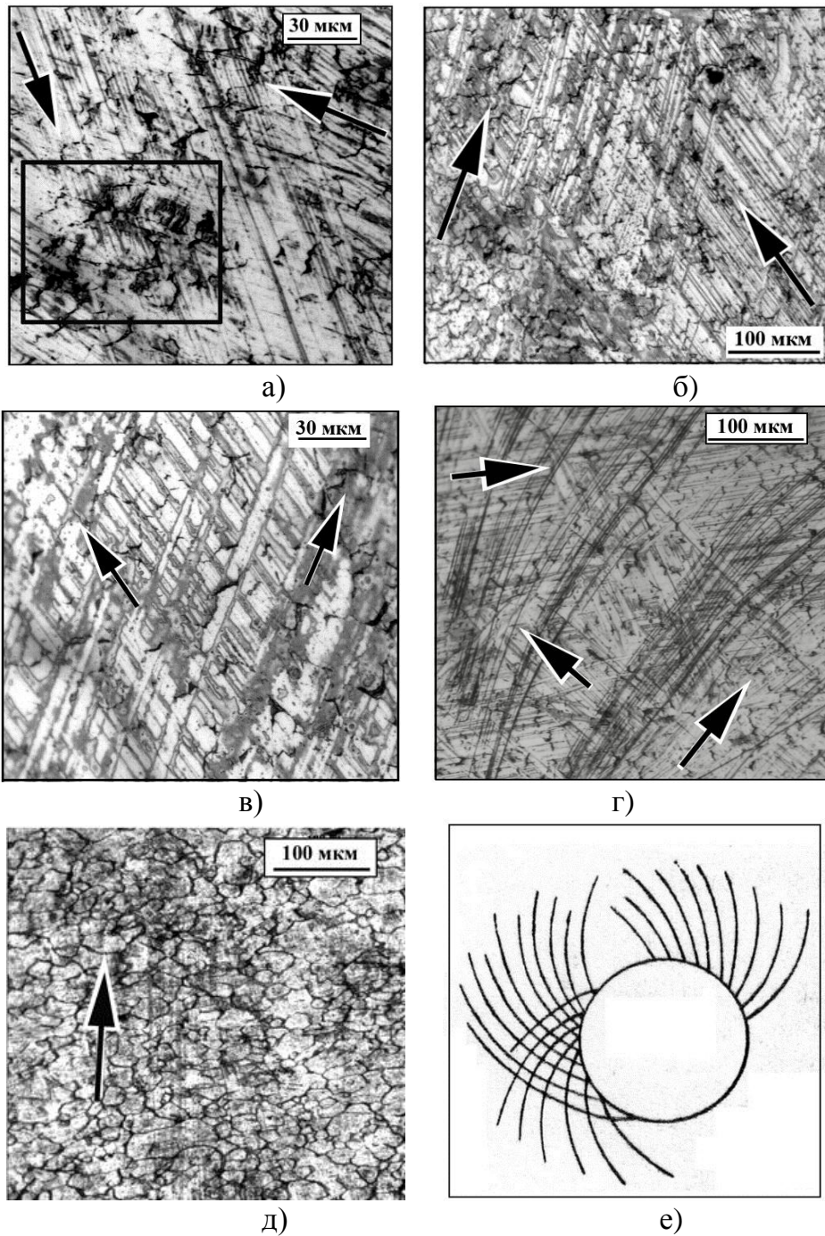
Рис. 5.6. Картины поверхностного слоя на образцах из стали ВНС9-Ш после испытания на усталость: a, б - \sigma_{\max} = 1300 МПа, N = 3 \cdot 10^3 циклов; в, г - \sigma_{\max} = 1300 МПа, N = 6 \cdot 10^3 циклов; д - \sigma_{\max} = 1300 МПа, N = 1,3 \cdot 10^4 циклов; е - полосы скольжения в стали у отверстия [49]. Стрелками указано направление полос сдвига.
