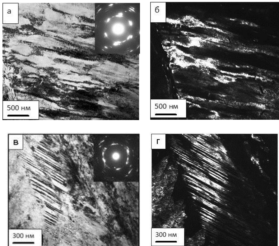
Рис.3.3. Микроструктура аустенита в деформированной структуре стали ВНС-9Ш: а - светлопольное изображение аустенита в рефлексе (200)- \gamma ; б - темнопольное изображение аустенита аустените в рефлексе (200)- \gamma ; в – светлопольное изображение двойников в аустените: г - темнопольное изображение двойников в аустените в рефлексе (111) - \gamma ;
