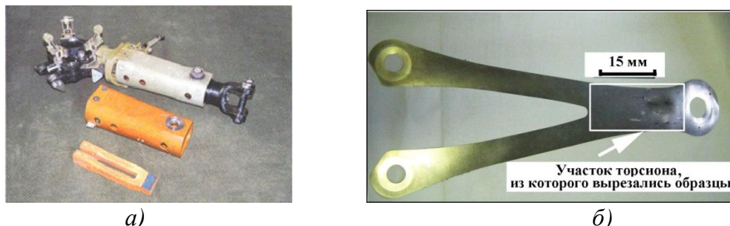
Рис. 5.21. Конструкция устройства [рукава] торсионного крепления лопасти вертолета к втулке несущего винта (а) [95] и зона вырезки материала, из торсионов после их эксплуатации (б).
