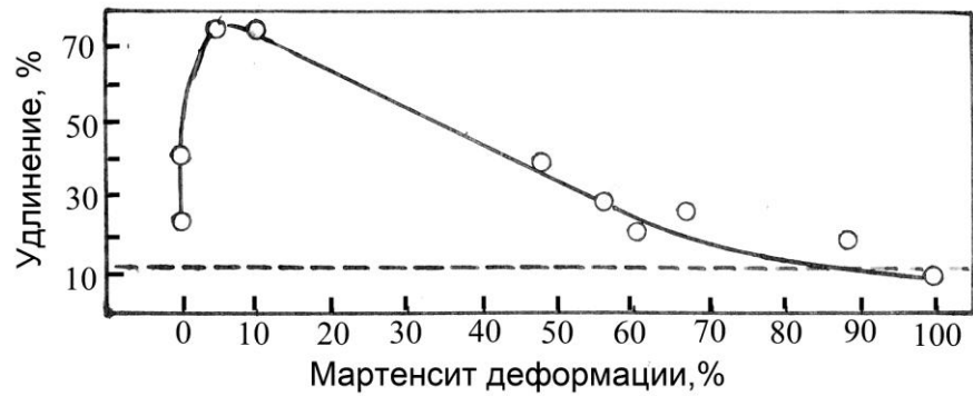
Рис. 6.4. Зависимость относительного удлинения от содержания мартенсита деформации в стали ВНС9-Ш (пунктирная линия отражает уровень минимального удлинения необходимого по ТУ)
