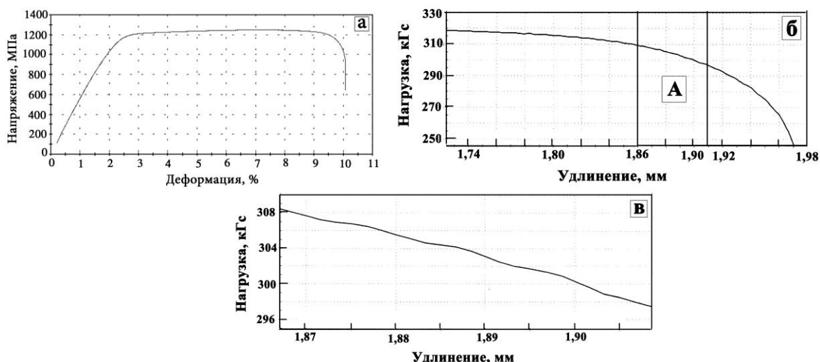
Рис. 4.2. Кривая растяжения трип – стали ВНС9-Ш при скорости деформирования 8,3 \cdot 10^{-5} \text{ с}^{-1} : а – общий вид кривой растяжения; б, в – детали кривой растяжения на стадии долома в области А.
