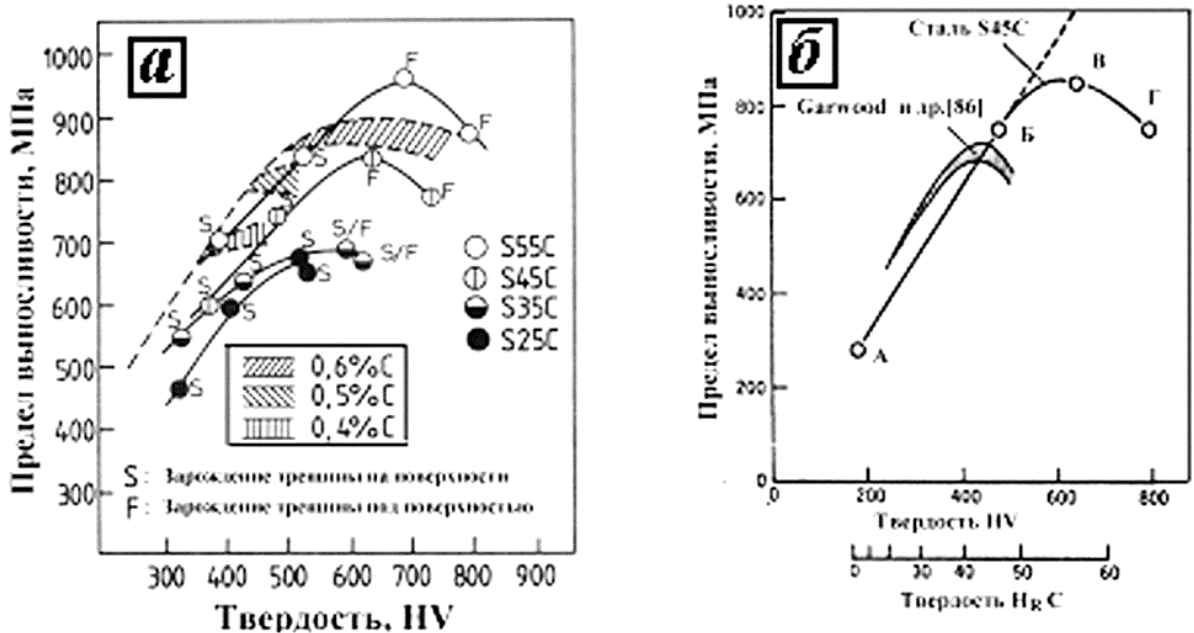
Рис. 1.4. Зависимость \sigma_R от твердости для ряда высокопрочных сталей: а – закаленных углеродистых высокопрочных сталей S55C (0,56%С, HV798, размер предшествующего аустенитного зерна d – 14 мкм); S45C (0,43%С, HV741, d – 13 мкм); S35C (0,33%С, HV625, d – 14 мкм); S25C (0,24%С, HV535, d – 17 мкм); [16]; б – углеродистой стали S45C с различным уровнем прочности (А – \sigma_B = 631 МПа, HV = 180; Б – \sigma_B = 1510 МПа, HV = 480); в – \sigma_B = 1962 МПа, HV = 650; з – \sigma_B = 2360 МПа, HV = 800) [17] и данных углеродистых сталей 0,4/0,45%С [18].
