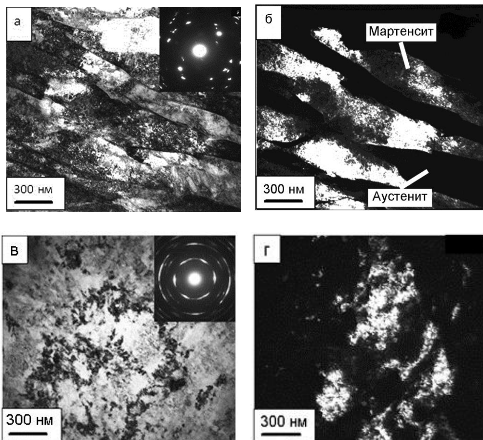
Рис. 3.2. Микроструктура мартенсита деформации в исходной структуре стали ВНС-9Ш: а - светлопольное изображение мартенсита деформации в рефлексе (200)- \alpha .; б - темнопольное изображение мартенсита в рефлексе (200)- \alpha .; в - светлопольное изображение мартенсита; г - темнопольное изображение мартенсита в рефлексе (100)- \alpha .
