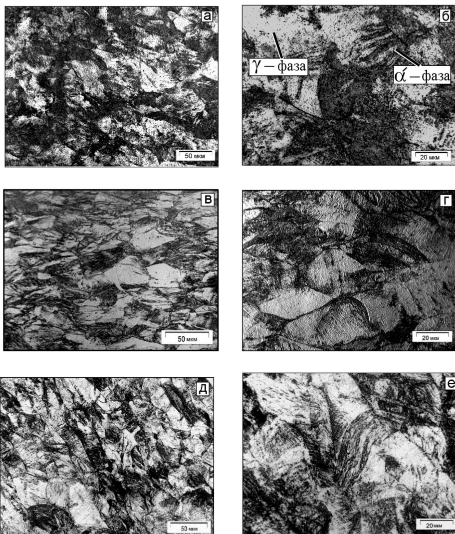
Рис. 4.11. Структура стали ВНС9-Ш (серия 2) после различных режимов отпуска: а, б –исходное состояние; в, г – 450 0 С; д, е - 600 0 С (оптическая микроскопия).
