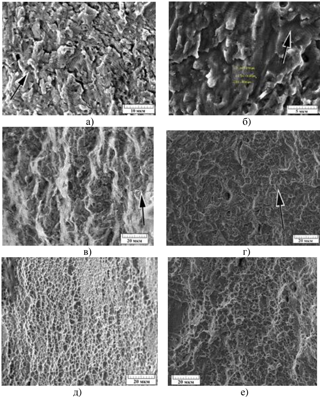
Рис. 5.7. Фрактография поверхности усталостного разрушения образцов из стали ВНС9-III: а, в, д - \sigma_{\max} = 925 МПа; б, г, е - \sigma_{\max} = 1700 МПа. Стрелками указано направление развития усталостной трещины.
