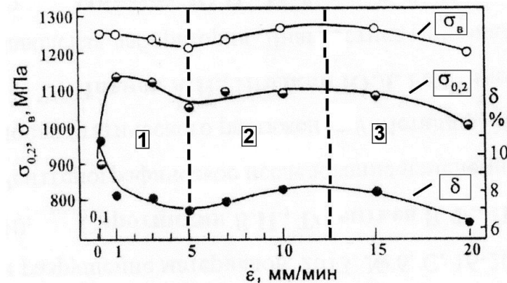
Рис. 4.6. Влияние скорости деформирования на изменение механических свойств стали ВНС9 –III серии 3.
