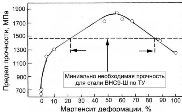
Рис. 6.1. Зависимость предела прочности от содержания мартенсита деформации в стали ВНС9-Ш
