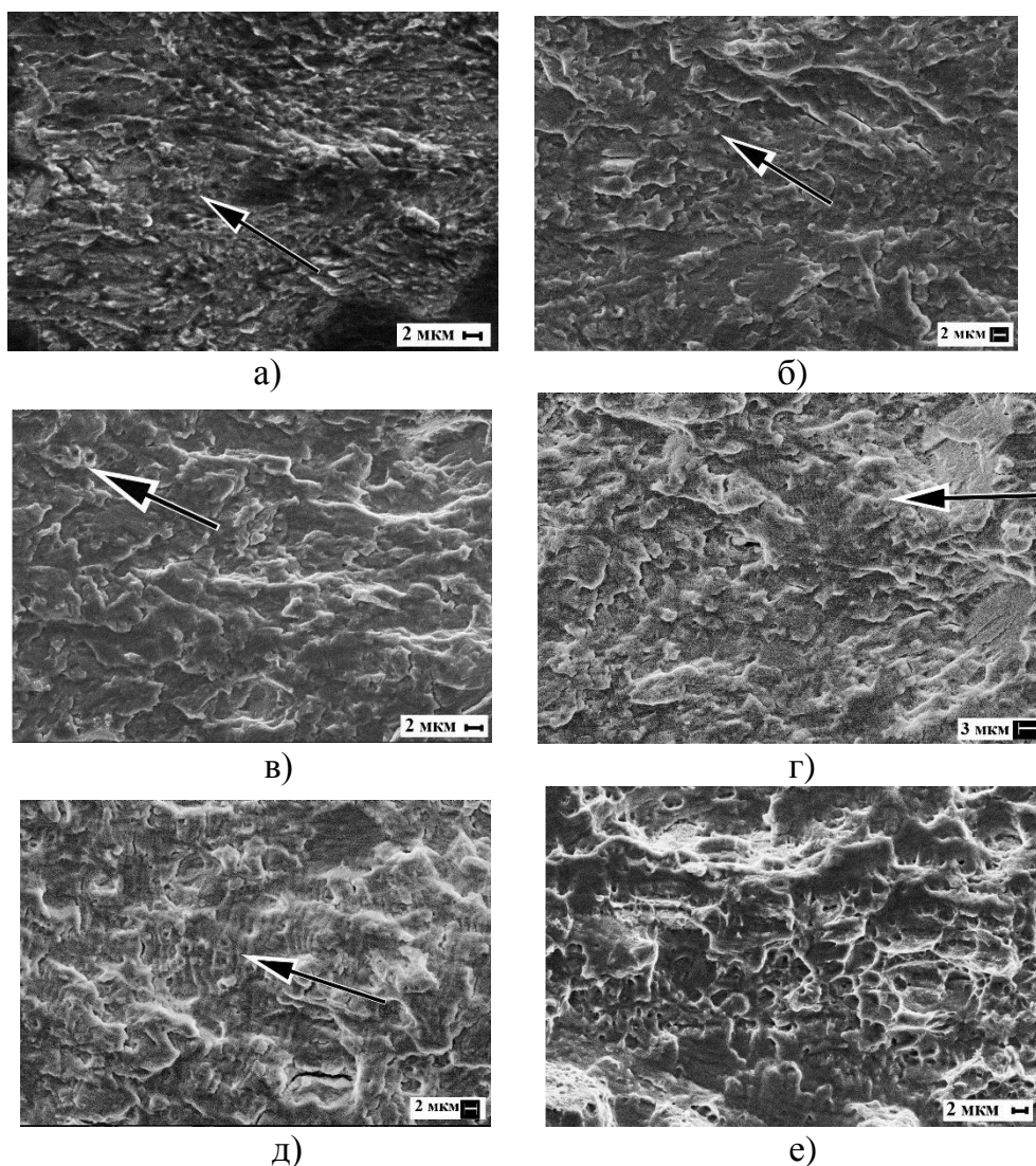
Рис. 5.21. Фрактография усталостного разрушения образцов типа II, вырезанных гидроабразивной резкой: а – \sigma_{\max} = 625 МПа, N = 2,0 \cdot 10^5 циклов до разрушения; б – \sigma_{\max} = 700 МПа, N = 8,5 \cdot 10^4 циклов; в – \sigma_{\max} = 625 МПа, N = 2,0 \cdot 10^5 циклов до разрушения; г – \sigma_{\max} = 700 МПа, N = 8,5 \cdot 10^4 циклов; д – \sigma_{\max} = 650 МПа, N = 3,0 \cdot 10^5 циклов; е – \sigma_{\max} = 625 МПа, N = 2,0 \cdot 10^5 циклов до разрушения.
