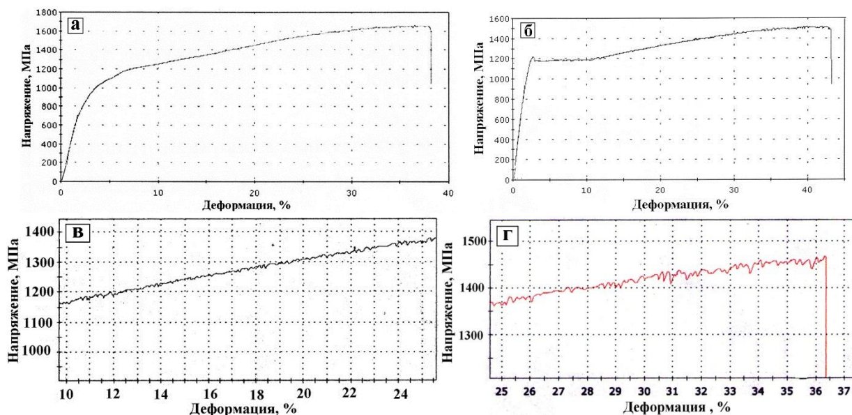
Рис. 5.23. Кривые статического растяжения образцов из трип – стали ВНС 9-Ш: а – образец из исходной ленты партии 1; б – образец, вырезанный из торсиона партии 2; в – участок кривой деформационного упрочнения торсиона партии 2 в интервале деформаций от 10 до 24%; г - участок кривой деформационного упрочнения торсиона 7 в интервале деформаций от 25% до окончательного разрушения.
