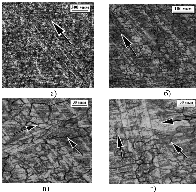
Рис. 5.4. Картины поверхностного слоя на образцах из стали ВНС9-Ш после испытания на усталость при \sigma_{\max} = 1700 МПа, N = 200 циклов. Стрелками указано направление полос сдвига.
