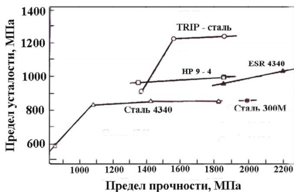
Рис. 1.6. Зависимость \sigma_R высокопрочных сталей от уровня предела прочности [20].
