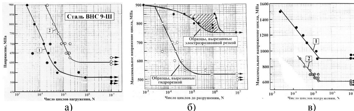
Рис. 5.17. Кривые усталости образцов из холоднокатаной ленты стали ВНС9-III: а) образцы, вырезанные гидроабразивной резкой: 1 образцы типа I; 2 – образцы типа II; б) кривые усталости образцов типа I: 1-электроэрозионная резка: 2– гидроабразивная резка; в) кривые усталости образцов типа II: 1- электроэрозионная резка: 2 – гидроабразивная резка.
