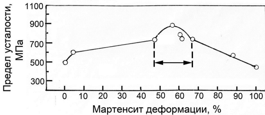
Рис. 6.5. Зависимость предела усталости от содержания мартенсита деформации в стали ВНС9-Ш.
