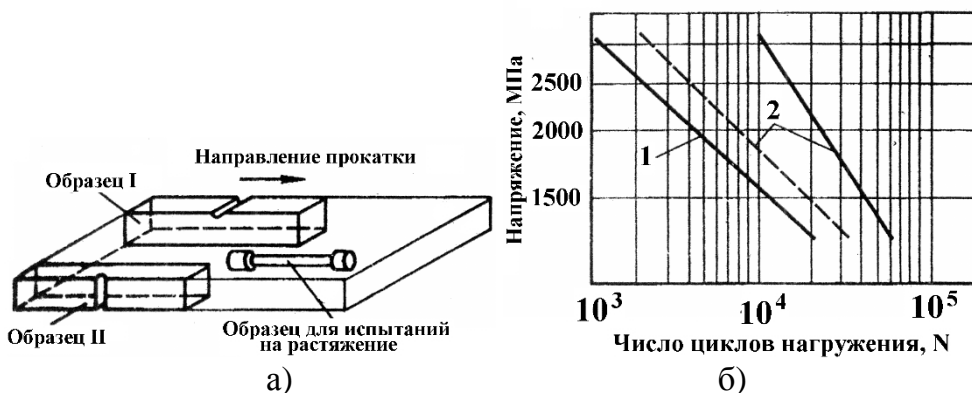
Рис. 1.11. Схема вырезки образцов (а) и кривые малоцикловой усталости сталей 30ХН2МФА (1) и 36Х9НМ4ГС2 (2); сплошные линии образцы типа I; штриховая линия – типа II (б) [23].
