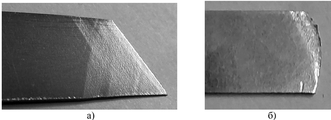
Рис.5.8. Макрокартина вида разрушения образца из стали ВНС9-Ш после статического растяжения (а) и после испытания на усталость (б) (x5).
