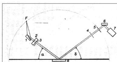
Рис. 3.9. Рентгенооптическая схема асимметричной съемки, реализованная на дифрактометре "Ultima IV". Ф - фокус рентгеновской трубки; ПЗ - параболическое зеркало; 1 - щели Соллера; 2 - щель, ограничивающая ширину падающего пучка рентгеновских лучей, 3 - щель, ограничивающая ширину дифрагированного пучка рентгеновских лучей; 4 - приемная щель; щель; М - плоский графитовый монохроматор; СД - сцинтилляционный детектор.
