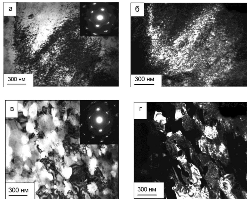
Рис. 4.16. Микроструктура феррита в стали ВНС9-Ш образцов серии 2 после отпуска при 650^{\circ}\text{C} : а - светлопольное изображение нерекристаллизованного феррита; б – темнопольное изображение в рефлексе (110) - \alpha ; в - светлопольное изображение рекристаллизованного феррита; г - темнопольное изображение в рефлексе (110) - \alpha .
