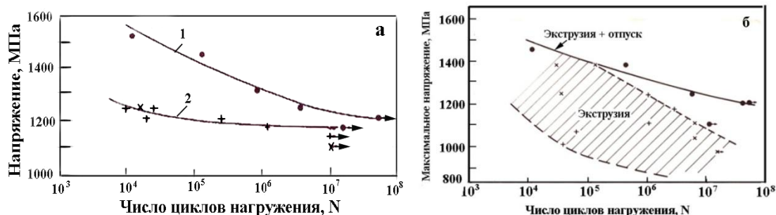
Рис. 1.5. Кривые усталости трип - стали [20]: а - после экструзии на 60% (1 – экструзия + отжиг; 2 – экструзия); б - после экструзии на 80% [20].
