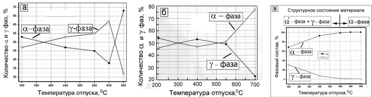
Рис. 4.15. Изменение количества \alpha - и \gamma - фаз образцов из стали ВНС9 – Ш в зависимости от температуры отпуска: а – рентгеновский анализ образцов, у которых выдержка при отпуске составляла 2 ч.; б – выдержка - 0,5 ч.; в – фазовый состав образцов (выдержка при отпуске 2 ч.), разрушенных при статическом растяжении.
