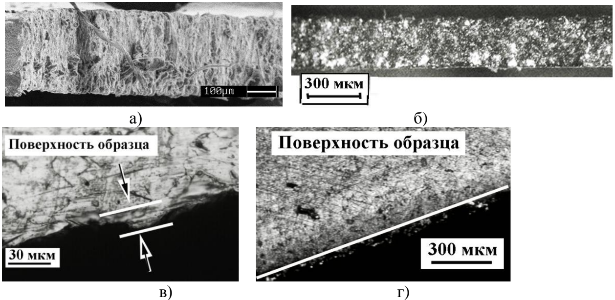
Рис. 5.18. Поверхность кромок образца, вырезанного различными методами: а – вид на боковую поверхность после гидроабразивной резки; б – вид на боковую поверхность после электроэрозионной резки в - профиль кромки реза после гидроабразивной резки; г - профиль кромки реза после электроэрозионной резки.
