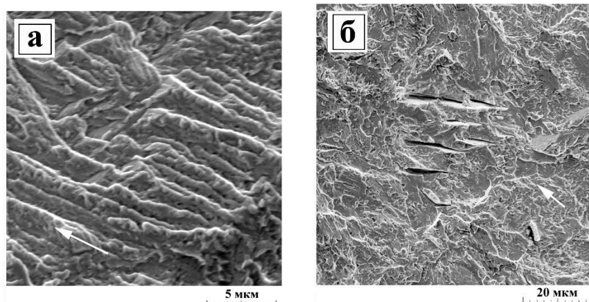
Рис. 1.10. Фрактография усталостного разрушения образца из трип – стали серии 3 ( \sigma_{\max} = 650 МПа, N = 6,5 \cdot 10^4 циклов); стрелками указано направление распространения трещины [22].
