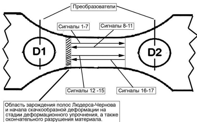
Рис. 3.21. Схема локализации сигналов АЭ в процессе статического растяжения образца из стали ВНС9-Ш на стадии деформационного упрочнения.
